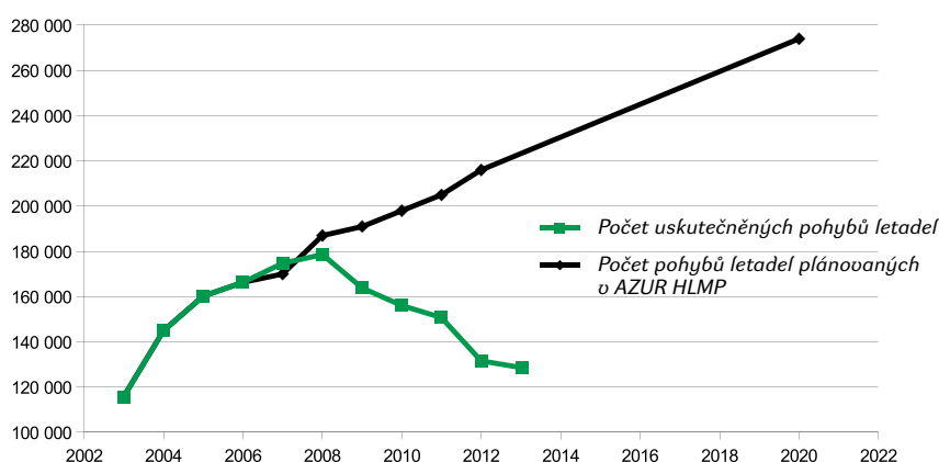
Počet uskutečněných a plánovaných pohybů (přistání/startů) letadel na letišti Praha-Ruzyně
